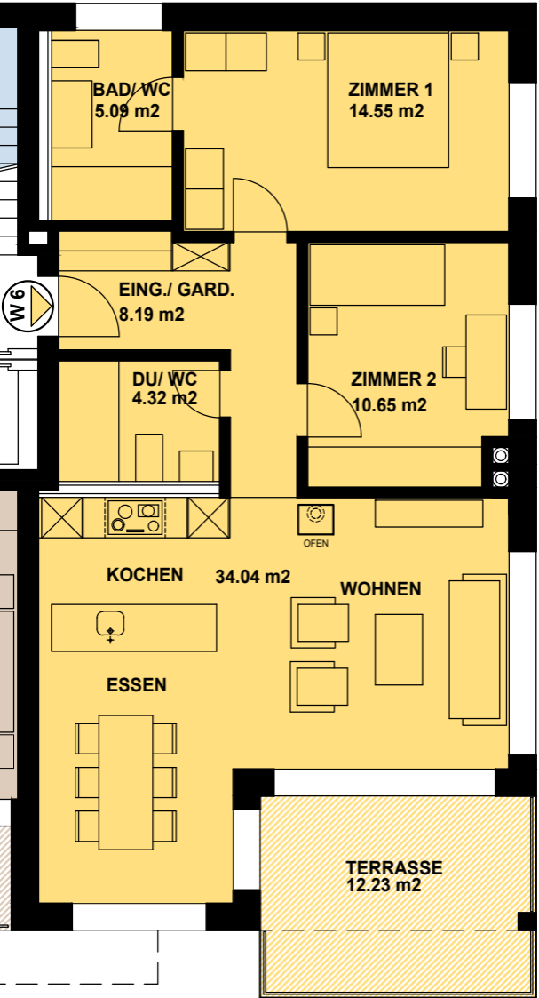
3 1/2 - ZIMMERWOHNUNG WF 83.03 m 2
