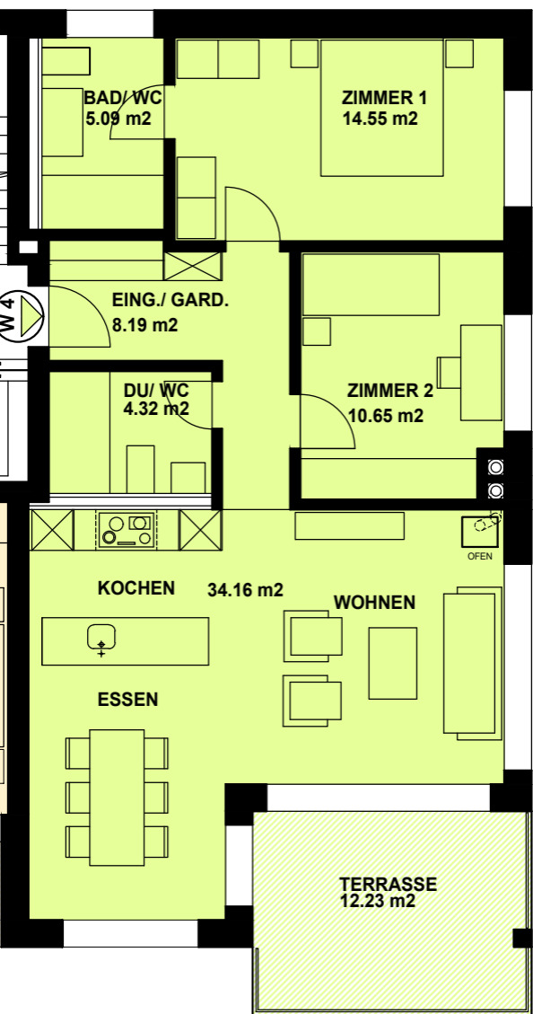
3 1/2 - ZIMMERWOHNUNG WF 83.17 m 2
